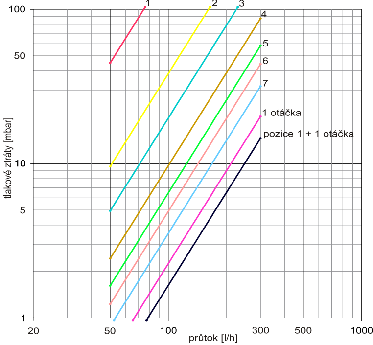
regulační ventil rozdělovače
